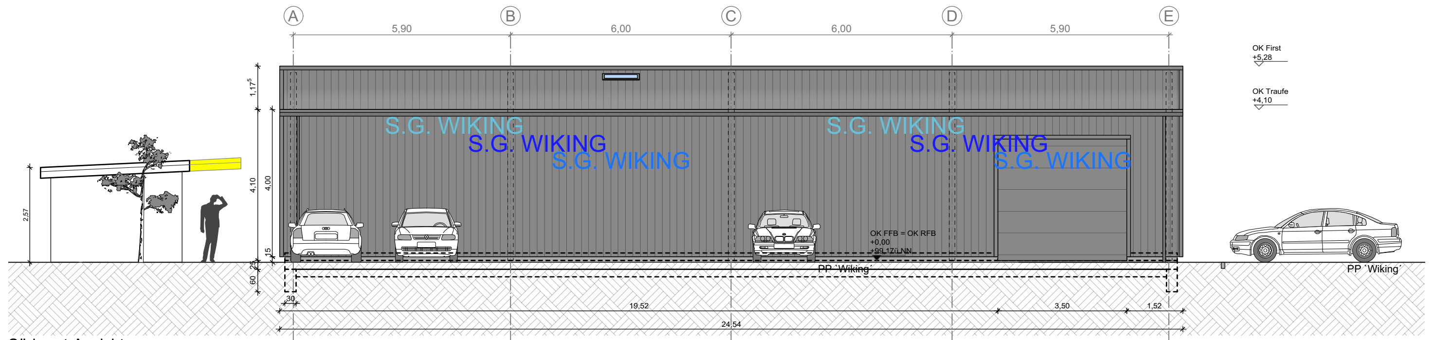
Südwest-Ansicht Sicht von der Straße zur Halle
